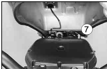
7. Connecteur de la sonde de niveau de carburant
