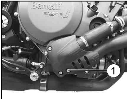
1. Aftapbout voor koelvloeistof
