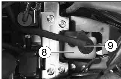
8. Koelvloeistofreservoir
