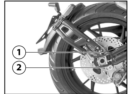
1. Rotor van het achterwiel 2. Sensor in het achterwiel
