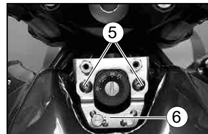
5. Schrauben (10 Nm festziehen) 6. Tankbefestigungsplatte
