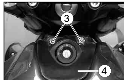
3. Schrauben (10 Nm festziehen) 4. Gummidichtung
