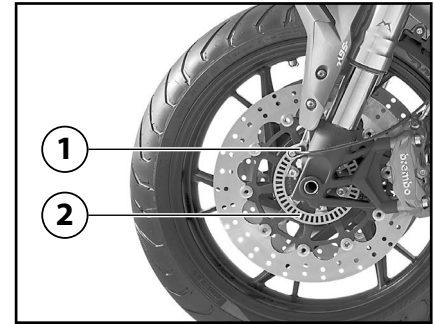
1. Sensor in het voorwiel 2. Rotor van het voorwiel
